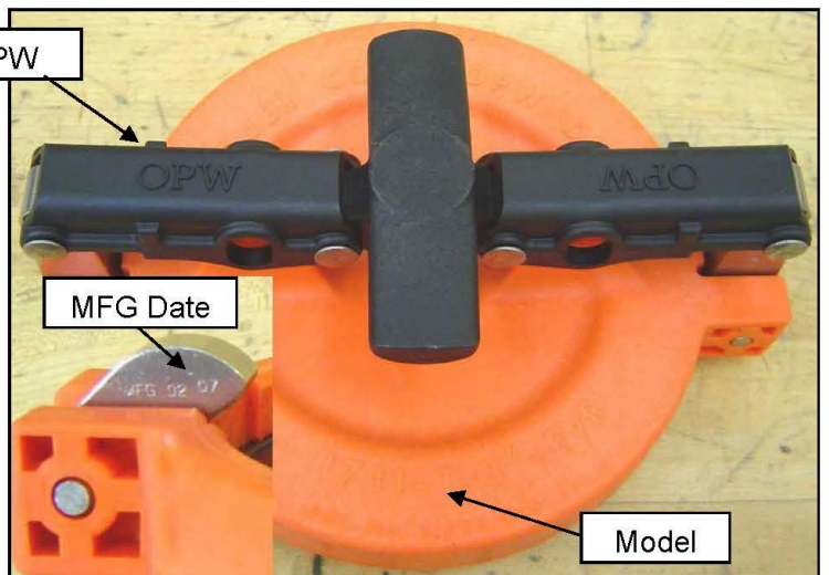
Figure 1-8 OPW 1711-T-EVR Vapor Dust Cap
